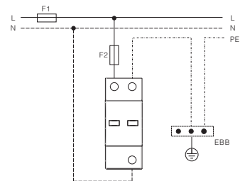
TT sústava - jednofázová 1+1 (T-zapojenie)
