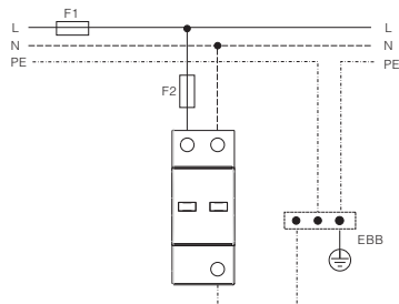
TT sústava - jednofázová 1+1 (T-zapojenie)
