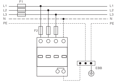
TT sústava - trojfázová 3+1 (T-zapojenie)
