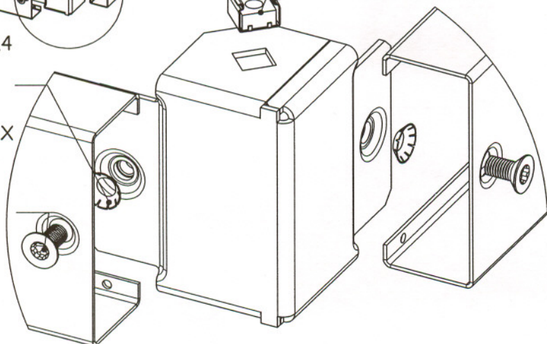
matice klecová M8
