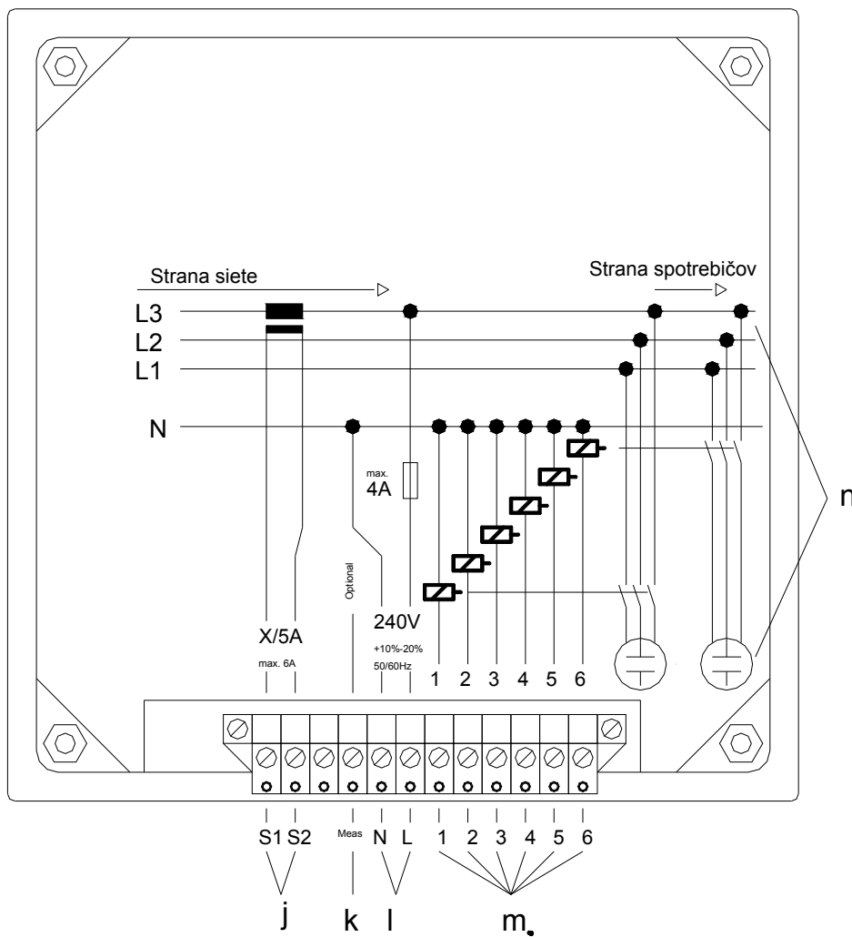
Obr. 2: Pohľad zozadu
