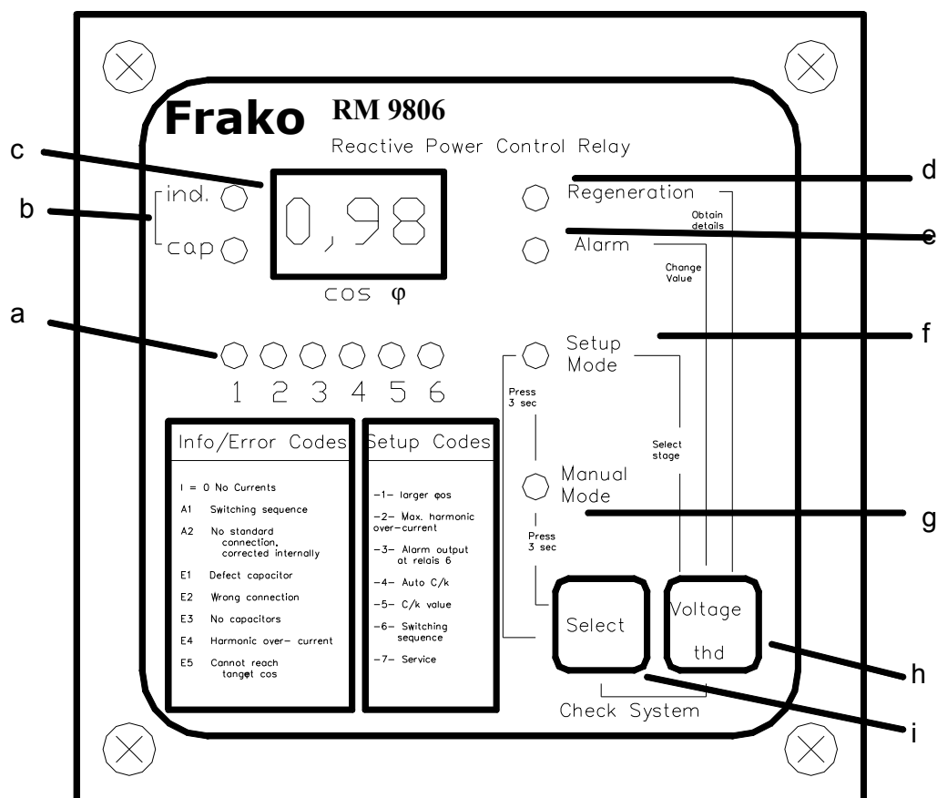
Obr. 1: Pohľad spredu
