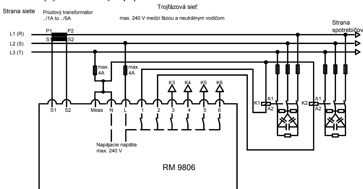
Obr. 6: Pripojenie v zvláštnych prípadoch
