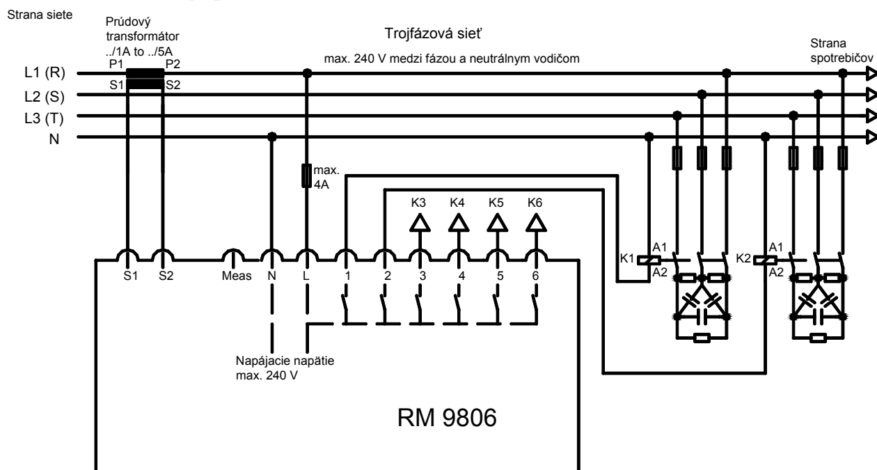
Obr. 3: Štandardné zapojenie
