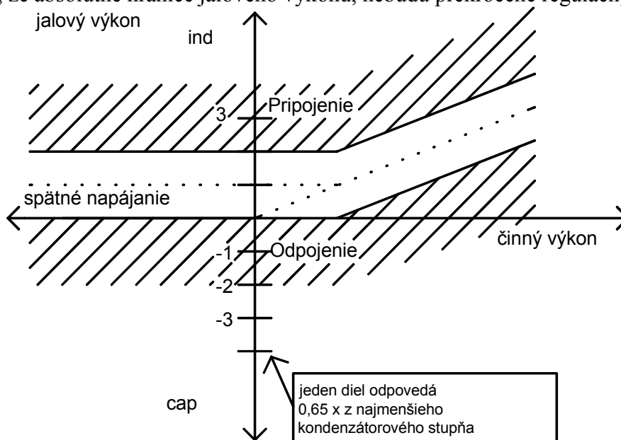
Obr. 8: Regulačné pásmo pri nastavení cieľového \cos \varphi = 0,92 ind; L = +1,0; PS = 0
