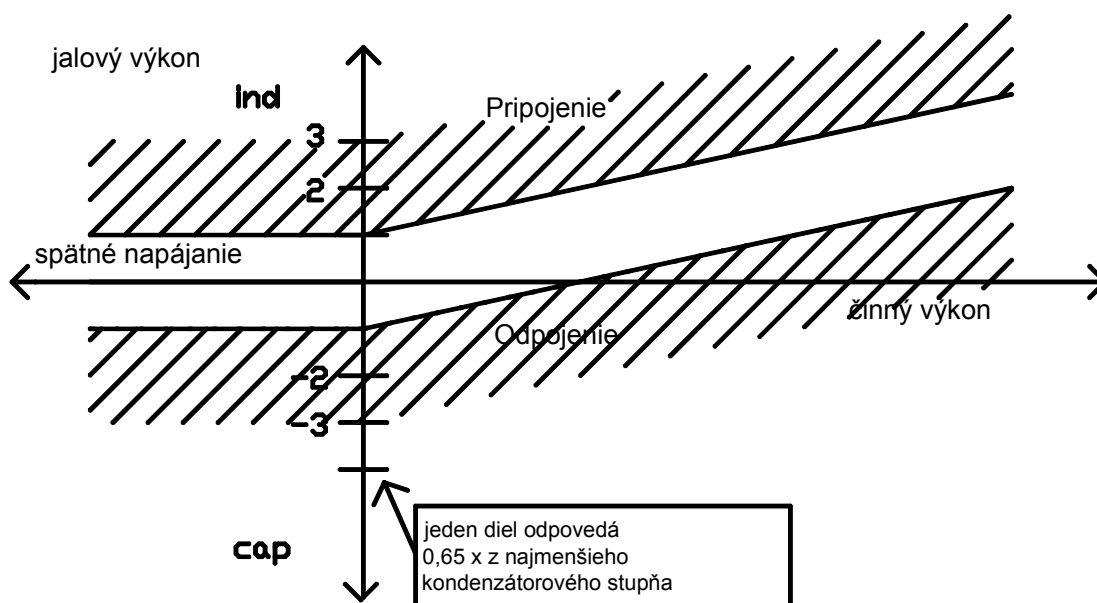
Obr. 5: Regulačné chovanie pri nastavení cieľového \cos \varphi = 0,92 ind.; L = OFF; PS = 0
