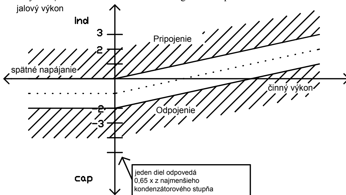
Obr. 7: Regulačné pásmo pri nastavení cieľového \cos \varphi = 0,92 ind; L = OFF; PS = -1,0
