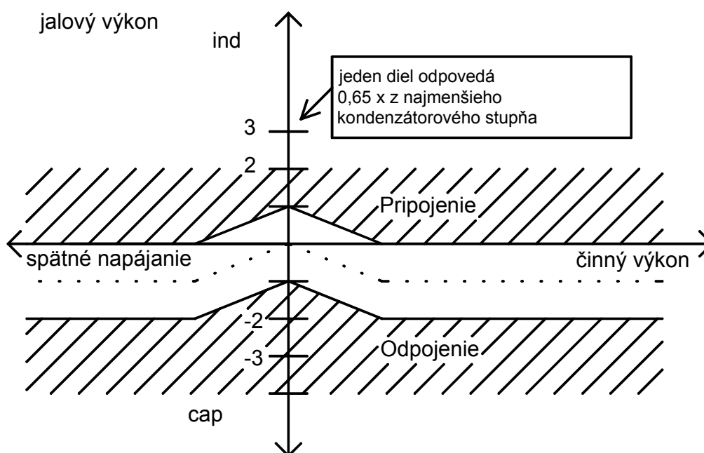
Obr. 9: Regulačné pásmo pri nastavení cieľového \cos \varphi = 0,92 ind; L = 1,0 ; PS = 0
