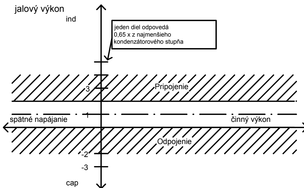
Obr. 6: Regulačné pásmo pri nastavení cieľového \cos \varphi = 1 ; L = OFF; PS = +1,0
