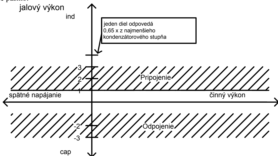
Obr. 4: Regulačné chovanie pri nastavení cieľového \cos \varphi = 1 ; L = OFF; PS = 0
