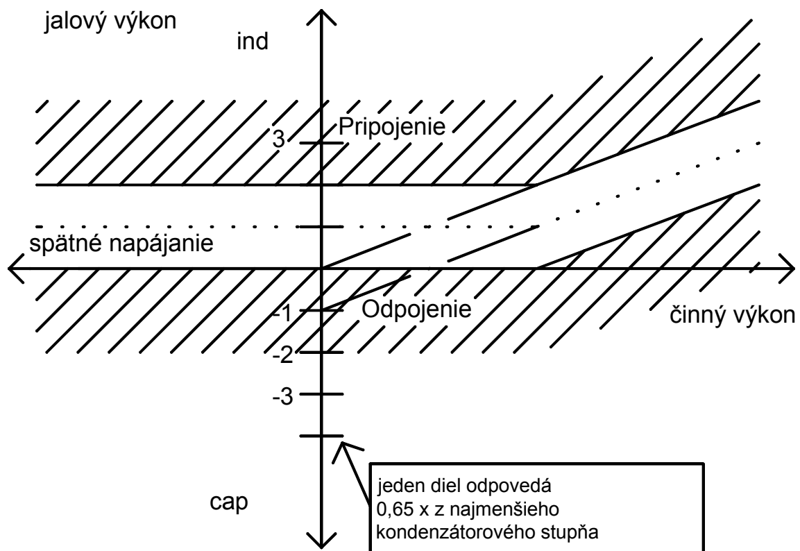
Obr. 9: Regulačné pásmo pri nastavení cieľového \cos \varphi = 0,92 ind; L = +1,0; PS = -1,0
