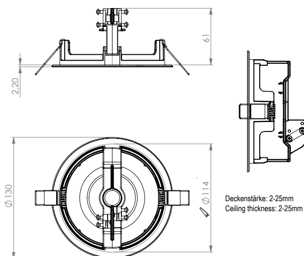
Rozmery zápusťného rámu NLILDE (mm)
